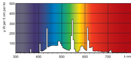
Barva světla typu TL-D de Luxe /965
