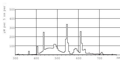
Barva světla typu TL-D de Luxe /965
