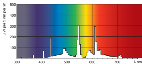
Barva světla typu TL-D de Luxe /940
