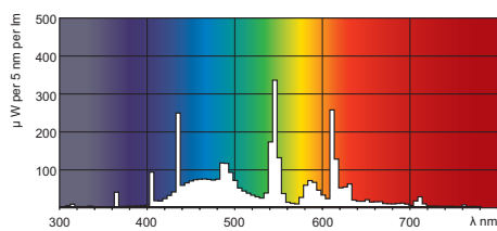
Barva světla typu TL-D de Luxe /965
