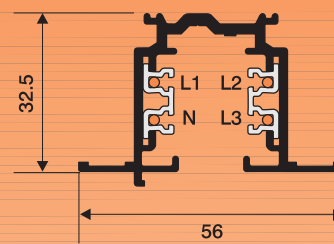
XTSF
